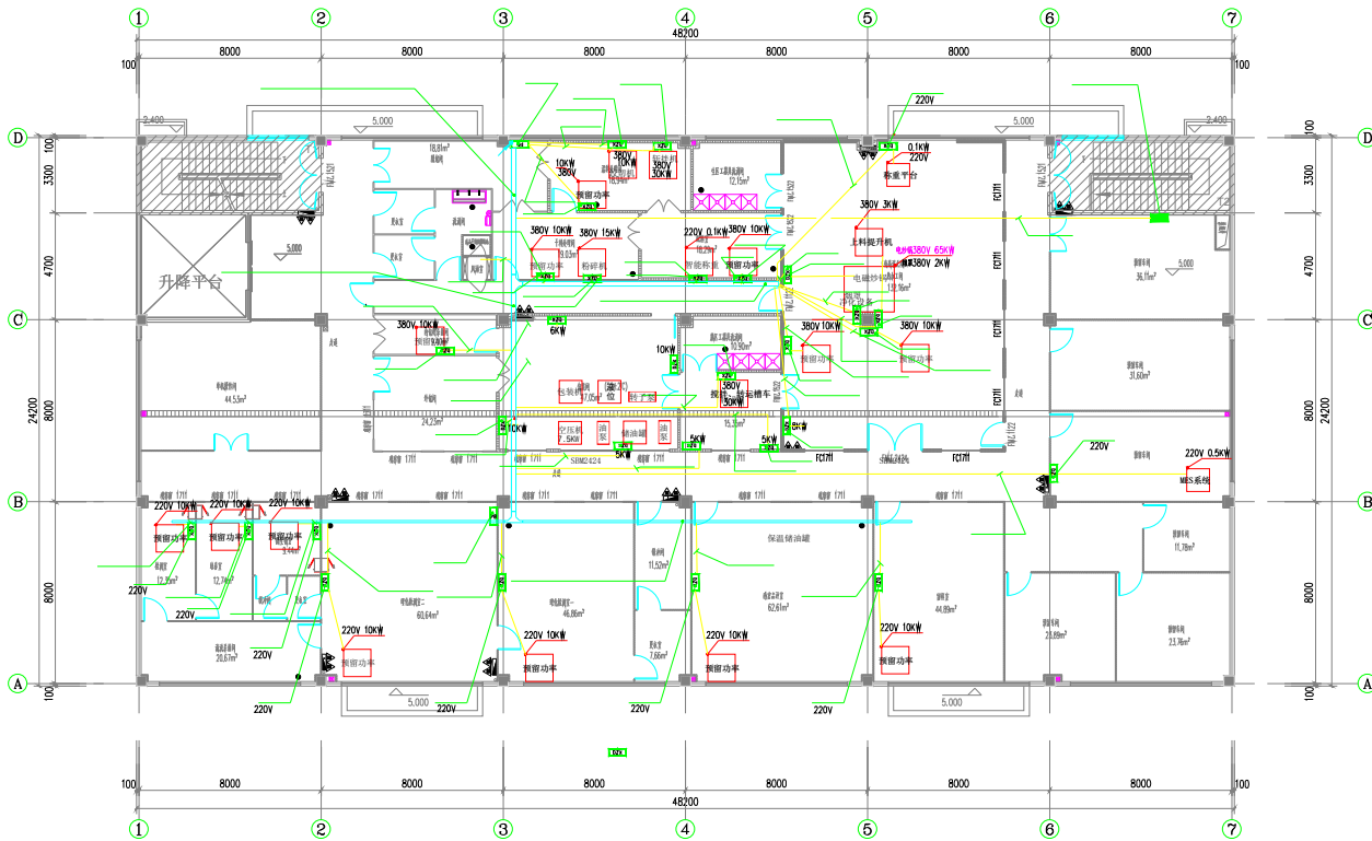
二层改造强电干线平面图 1:100
